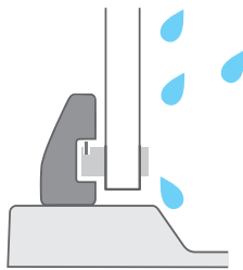
Rahmen im unteren Bereich der Kabine: Nexty, Pivot, Blix Slim, Blix, Objekt
